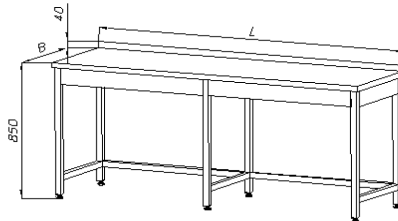
Art. Nr 1031 Arbeitstisch groß Aufkantung 40mm hinten inkl. ,links und rechts möglich ohne zzk
