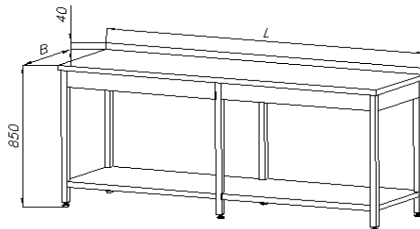
Art. Nr 1046 Arbeitstisch mit Boden x2 Aufkantung 40mm hinten inkl. ,links und rechts möglich ohne zzk
