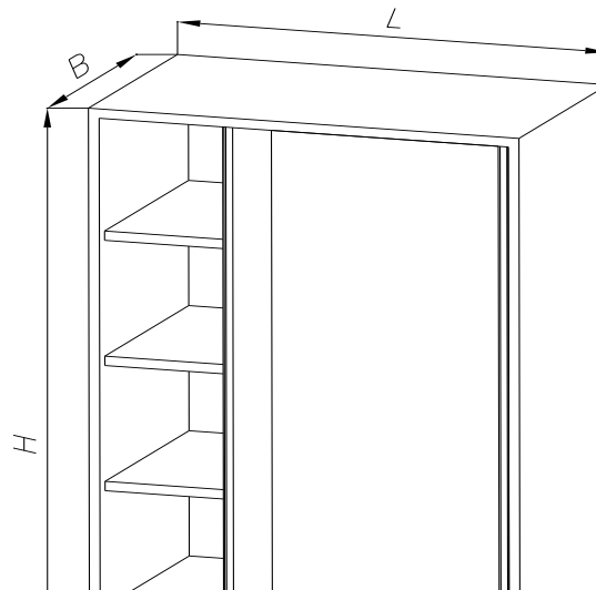
Art. Nr 3070 Durchlautschrank
