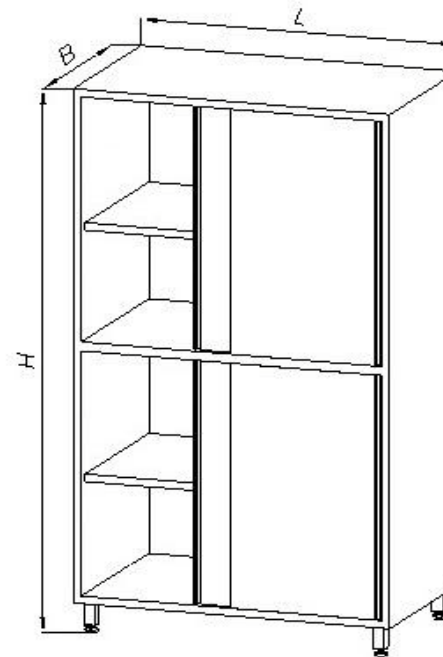
Art. Nr 3095 Durchlaufschrank
